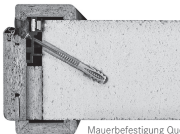
Mauerbefestigung Querschnitt
