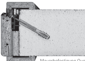
Mauerbefestigung Querschnitt
