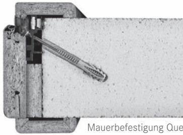
Mauerbefestigung Querschnitt
