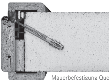
Mauerbefestigung Querschnitt
