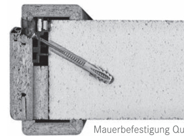
Mauerbefestigung Querschnitt
