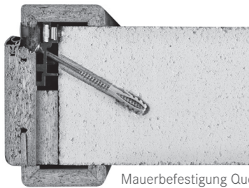
Mauerbefestigung Querschnitt
